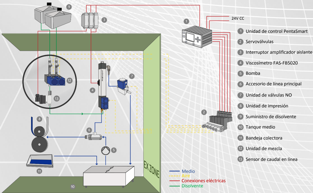
(Fig. S6-FB Sistema de control de la viscosidad con opción de mezcla para 2 disolventes)
